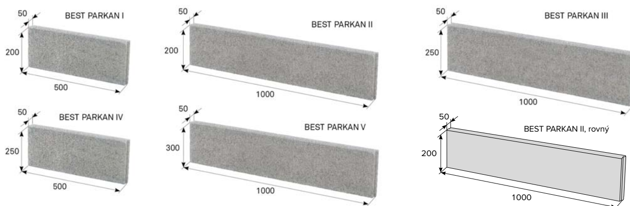
Skladebné rozměry
