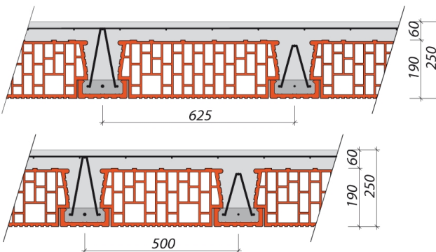
Tloušťka stropu 250 mm
