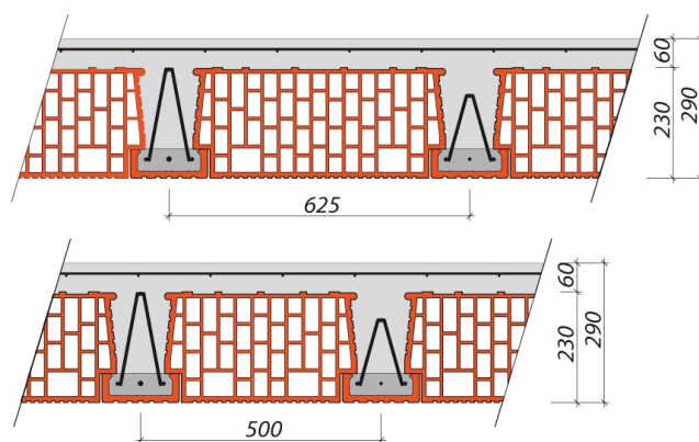
Tloušťka stropu 290 mm
