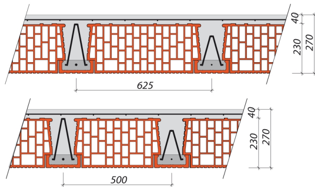
Tloušťka stropu 270 mm
