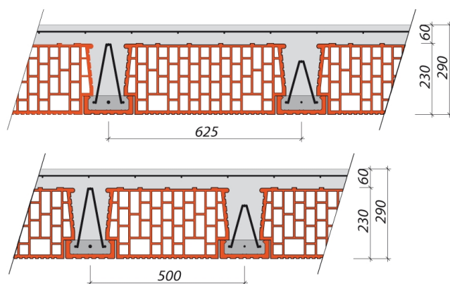
Tloušťka stropu 290 mm
