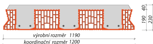
Panely PZU a balkonové - příčný řez panely šířky 1200 mm
