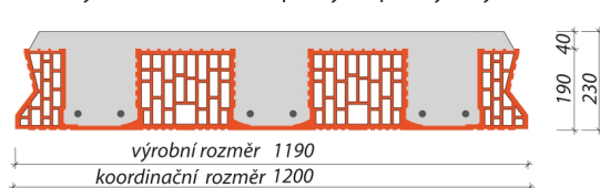
Panely PZU a balkonové - příčný řez panely šířky 1200 mm
