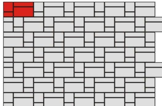
Obr. č.14 – Návrh skladby ze zdicích prvků History
