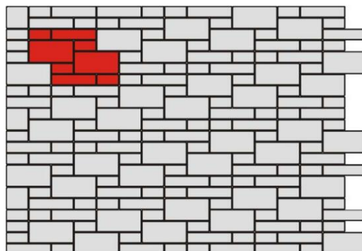
Obr. č.8 – Návrh skladby ze zdicích prvků History
