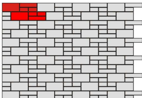
Obr. č.9 – Návrh skladby ze zdicích prvků History
