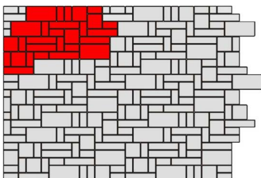
Obr. č.15 – Návrh skladby ze zdicích prvků History
