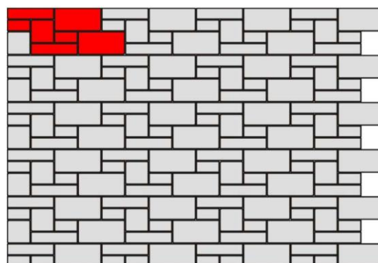
Obr. č.10 – Návrh skladby ze zdicích prvků History
