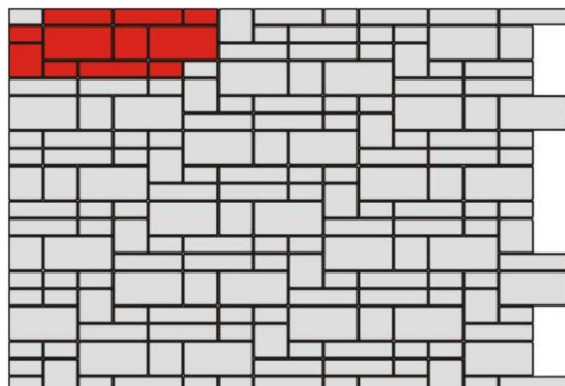
Obr. č.13 – Návrh skladby ze zdicích prvků History
