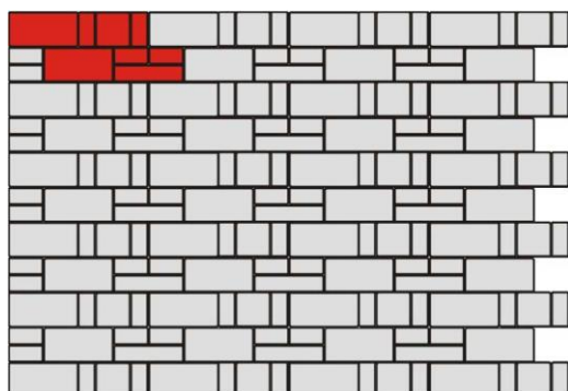
Obr. č.5 – Návrh skladby ze zdicích prvků History
