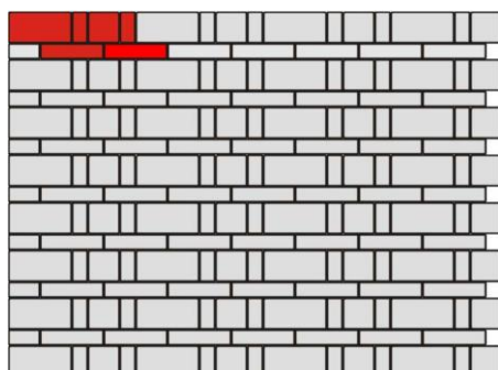
Obr. č.3 – Návrh skladby ze zdicích prvků History
